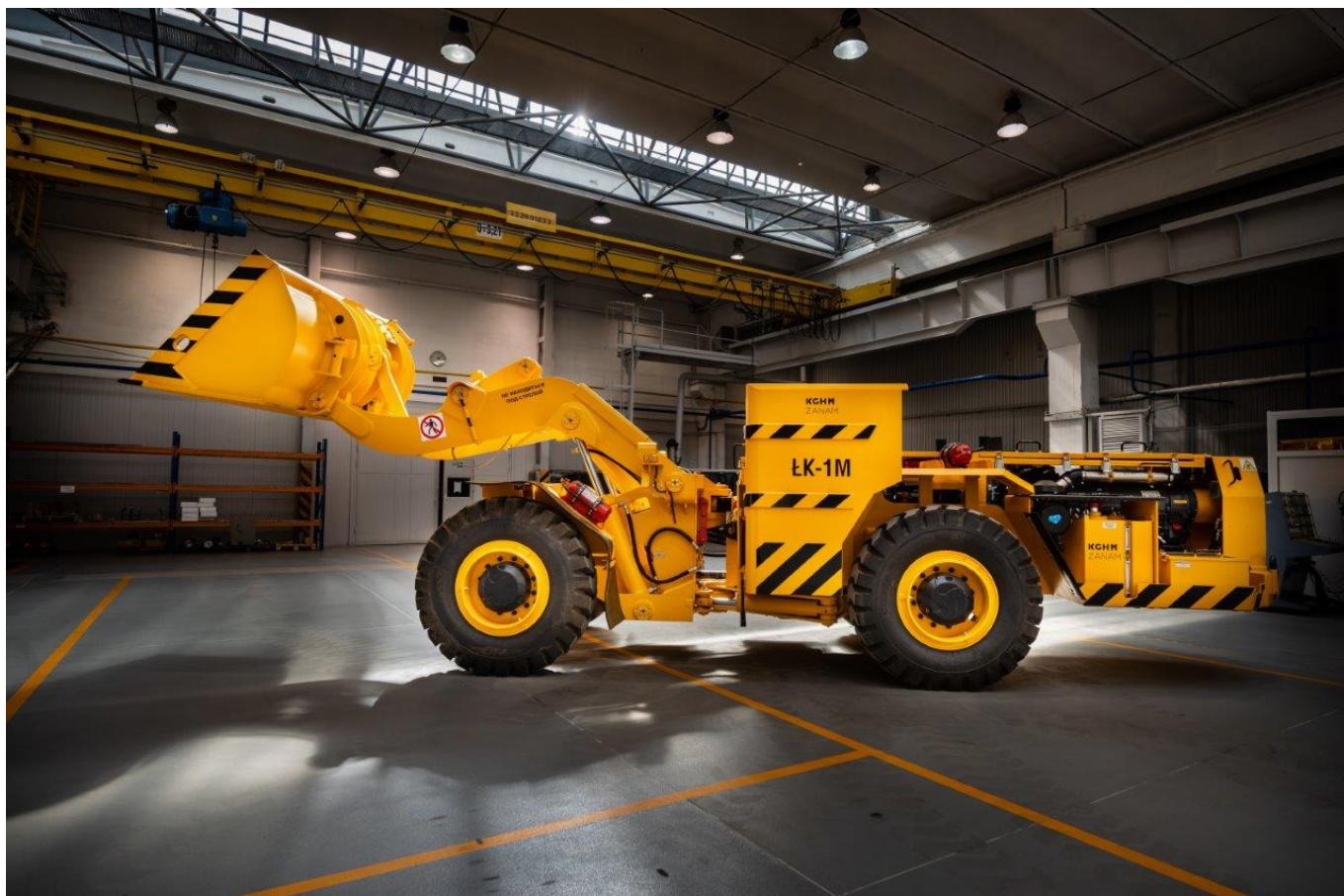
Ładowarka typu ŁK-1M
